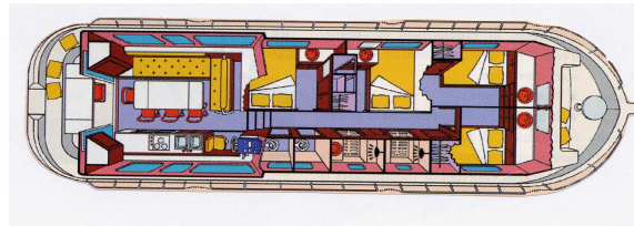
Coupe intérieure de la Pénichette 1500 R
